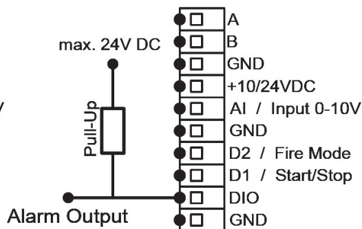
Připojení výstupu alarmu
