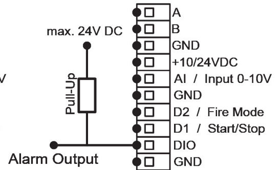
Anschluss Alarmausgang
