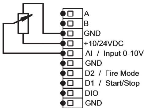
Anschluss Potentiometer
