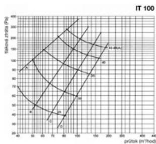
Otevření ventilu: A=1/4, B=1/2, C=3/4, D=1/1
