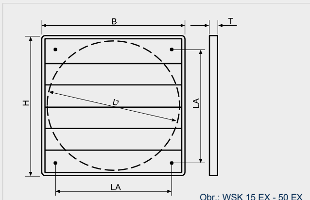
Obr.: WSK 15 EX - 50 EX
