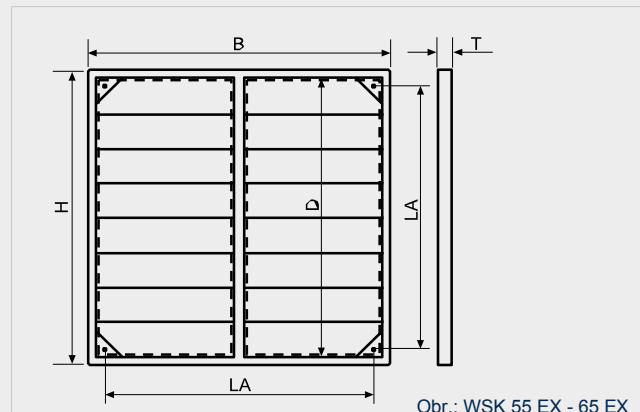
Obr.: WSK 55 EX - 65 EX
