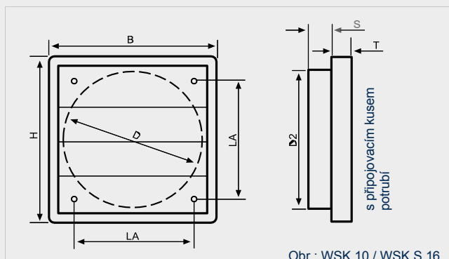
Obr.: WSK 10 / WSK S 16
