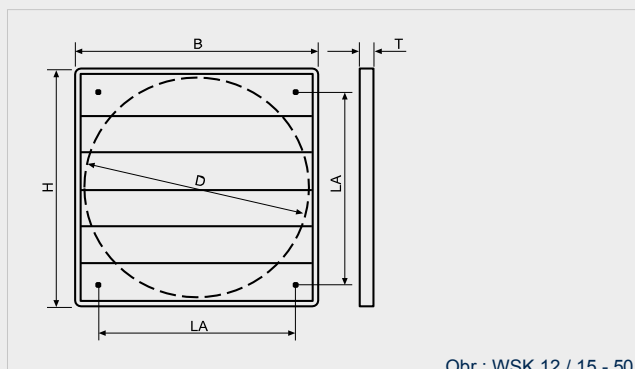
Obr.: WSK 12 / 15 - 50
