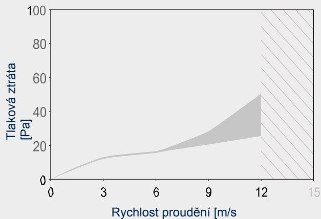
Tlakové ztráty WSK 15 -
