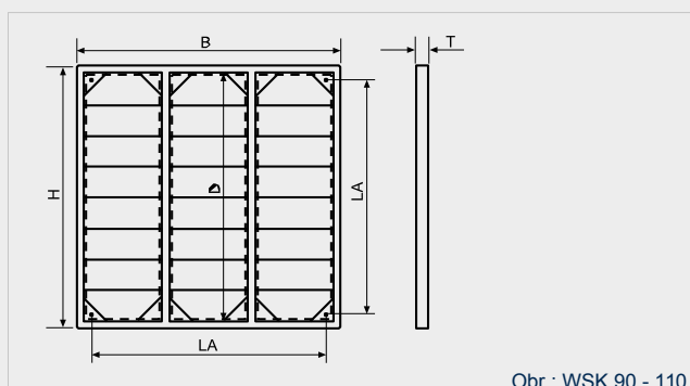
Obr.: WSK 90 - 110
