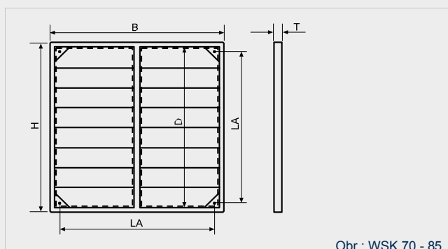
Obr.: WSK 70 - 85
