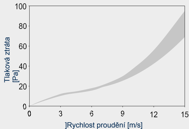
Tlakové ztráty WSK 55 - 110
