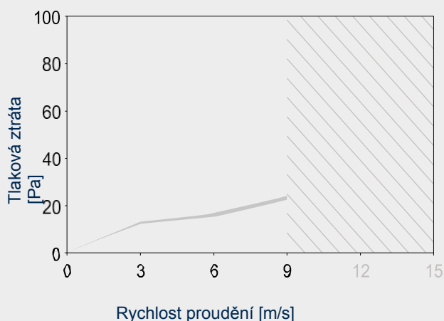
Tlakové ztráty WSK 15 -
