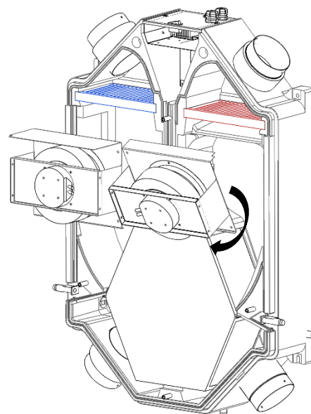
4) OTOČENÍ PODSESTAVY VENTILÁTORU PRO LEPŠÍ PŘÍSTUP
