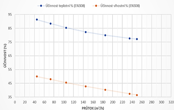
GRAF ÚČINNOSTI - XH2-30-ECS0ERxxS-0A0
